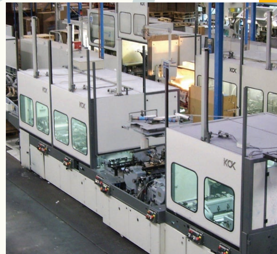
Modernste Hüllenfertigung auf W&D 202.00 High-Speed mit Inline-Qualitätskontrollsystem
