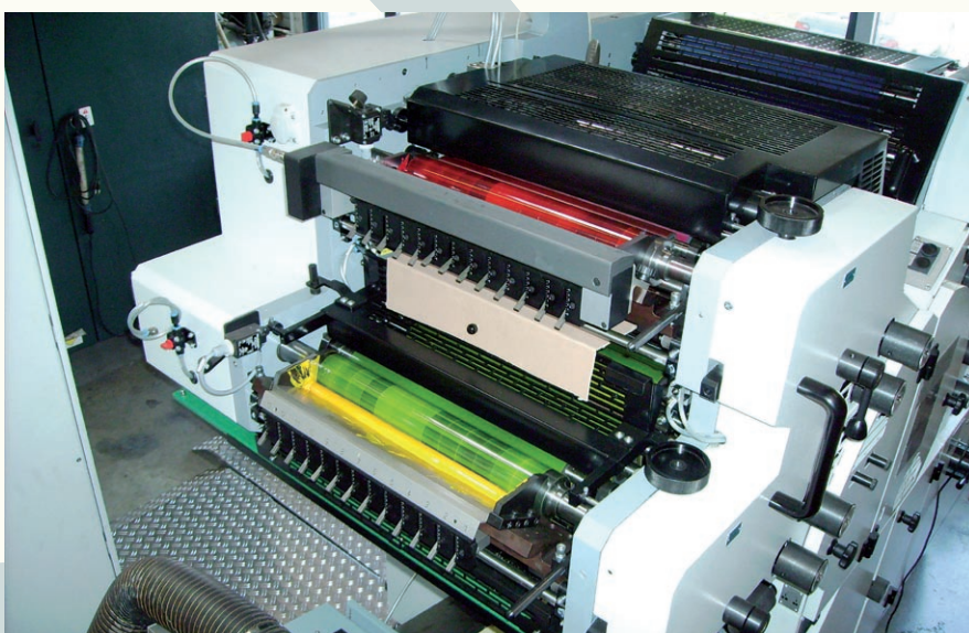
Detailansicht Druckwerk W&D 224
