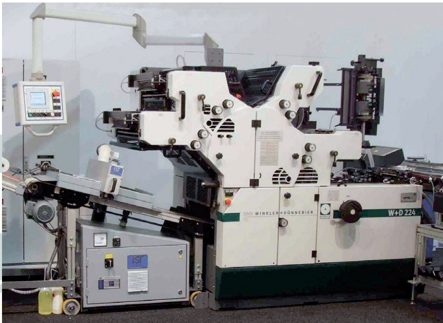
Vierfarb-Druckmaschine W&D 224 mit UV-Trocknung
